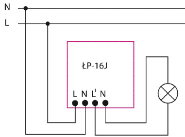
Czujnik ruchu
