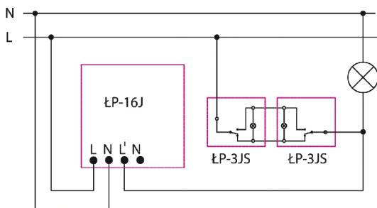
Czujnik ruchu + dwa łączniki zmienne
