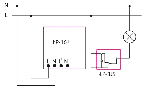
Czujnik ruchu + łącznik zmienny
