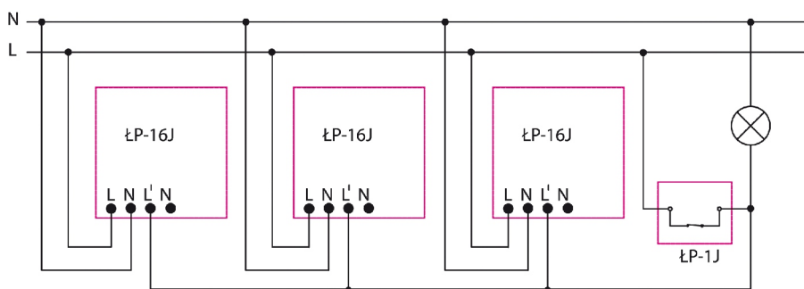
Dowolna liczba czujników + łącznik jednobiegunowy
