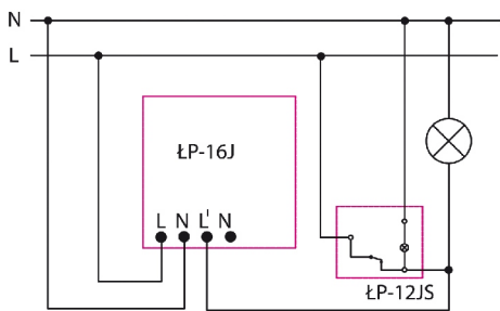
Czujnik ruchu + łącznik kontrolny
