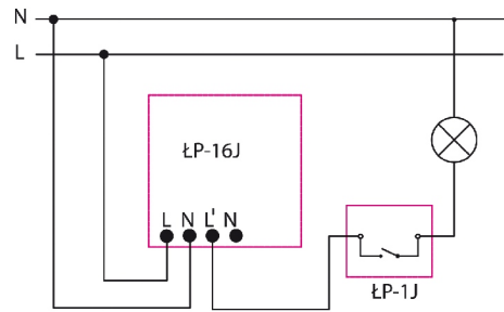
Czujnik ruchu + łącznik jednobiegunowy
