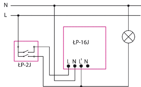
Czujnik ruchu + łącznik dwugrupowy
